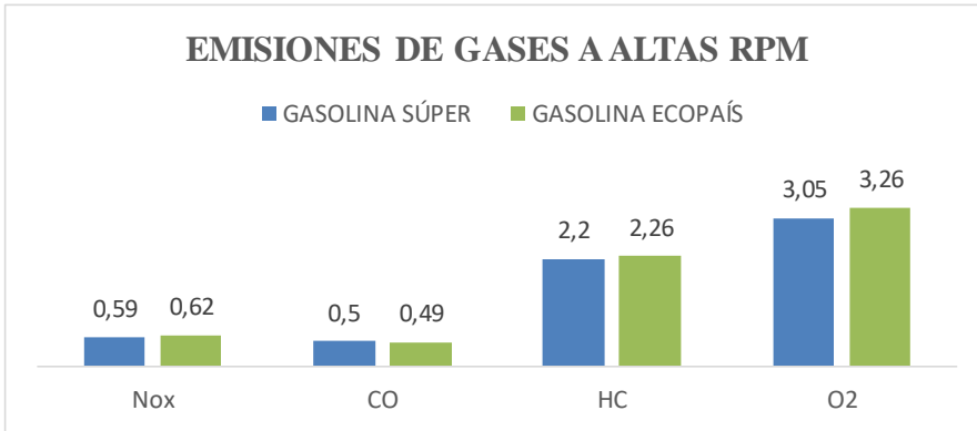
Figura 13. Emisiones de gases a altas rpm.
