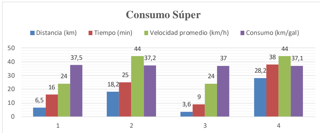
Figura 10. Distancia recorrida y consumo gasolina Súper.
