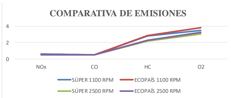
Figura 18. Emisiones de gases comparativas
