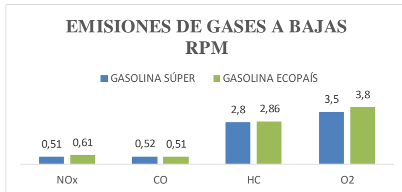
Figura 12. Emisiones de gases a bajas rpm.
