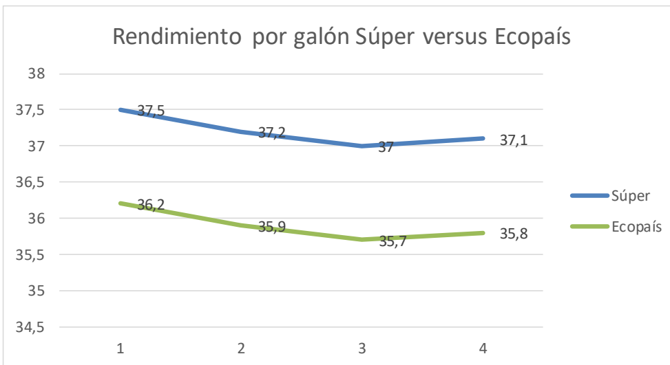
Figura 14. Comparativa del rendimiento Súper versus Ecopaís (km/gal).
